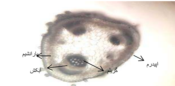
شکل ۱۷: ساقه شیدرک تیمار شده با غلظت ۷ میلی گرم در کیلوگرم سولفات مس (×۱۰)
