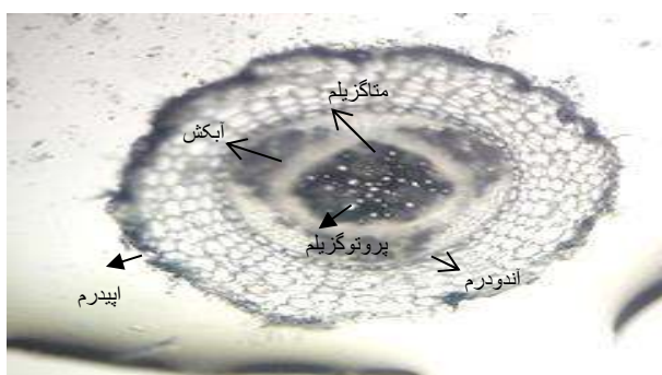
شکل ۳: ریشه شبدرک تیمار شده با غلظت ۱ میلی گرم در کیلوگرم سولفات مس (×۱۰)
