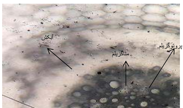
شکل ۴: آون های ریشه شبدرک تیمار شده با غلظت ۱ میلی گرم در کیلوگرم سولفات مس (×۴۰)
