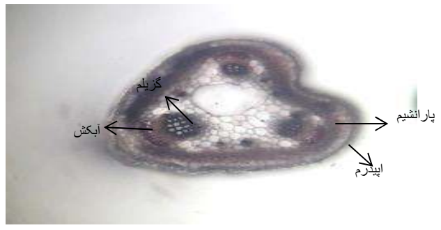
شکل ۱۹: ریشه شیدرک تیمار شده با غلظت ۴ میلی گرم در کیلوگرم سولفات مس (×۱۰)
